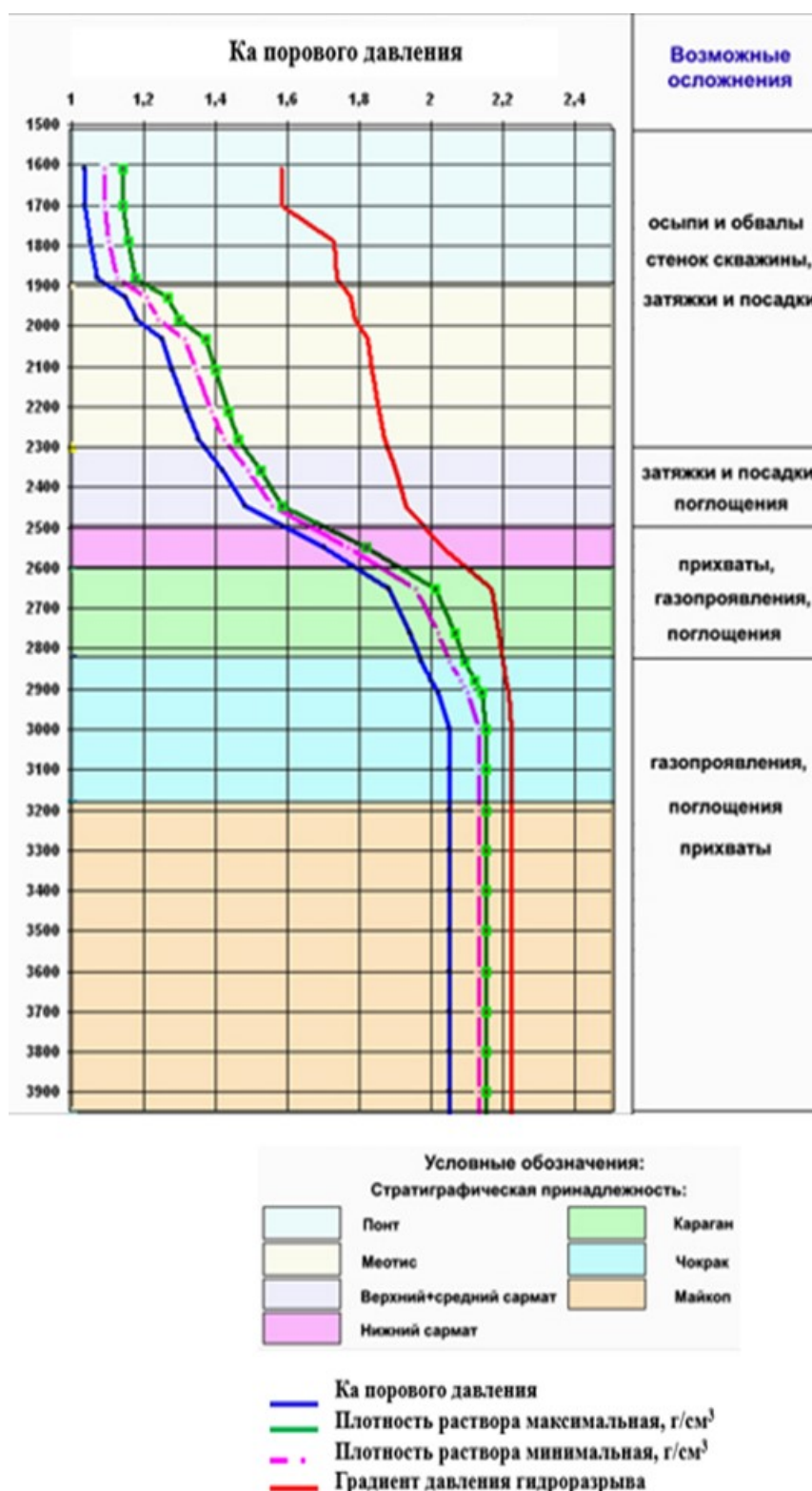
Рис. 4. График соотношения давлений для проекта строительства поисково-оценочной скважины в акватории Азовского моря
