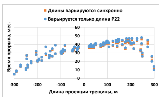
Рис. 10. График зависимости T от L_{np} при расчете упрощенным и базовым способами для скв. P22
